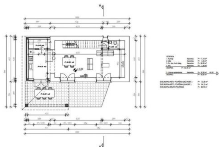
TLOCRT PRIZEML M 1:100
