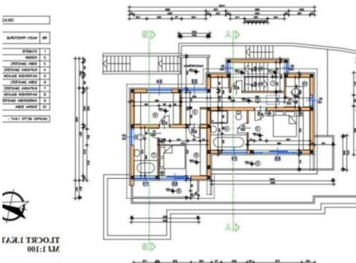
ПЛОСКИ ПРВ M 1:100
