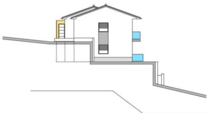
СЕВЕРНА ФА М1:100
