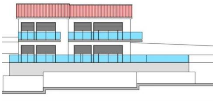
ИСТОЧНА ФАС М1:100
