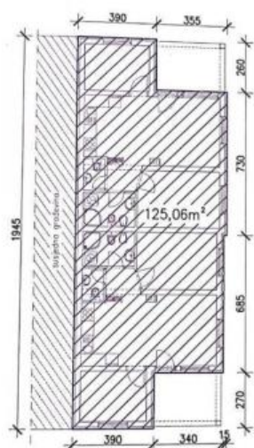
TLOCRT PRIZEMLJA
