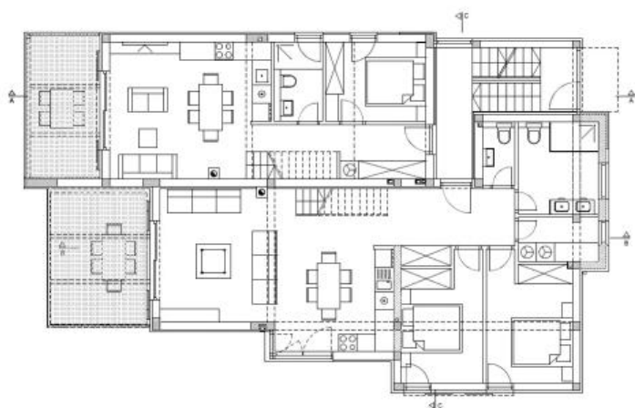
TLOCRT 2. KATA
