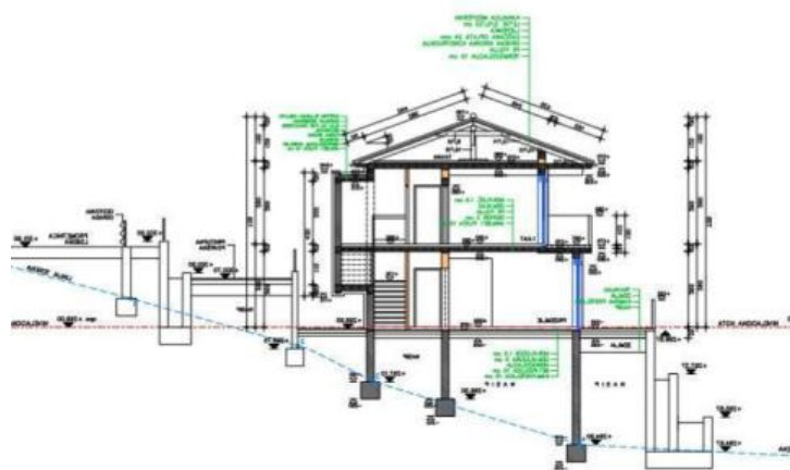
PRESEK M 1:100
