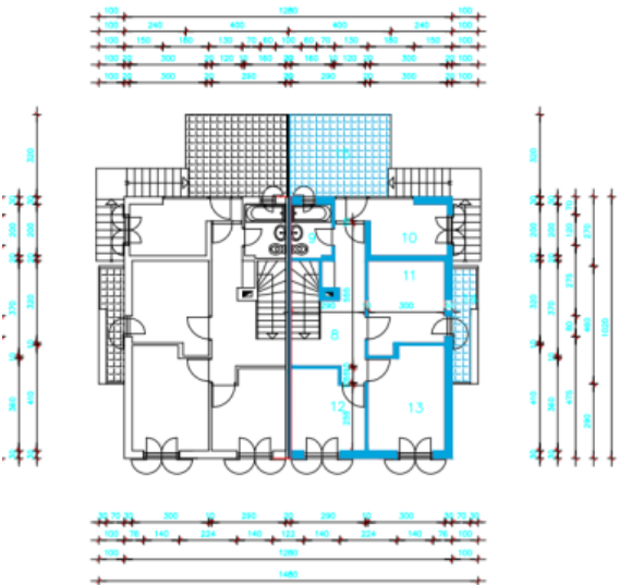
TLOCRT M 1:100
