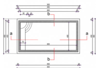
TLOCRT BAZENA (bruto površina 33,75m 2 )
