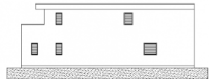
JUŽNO PROJEKLE 1:100
