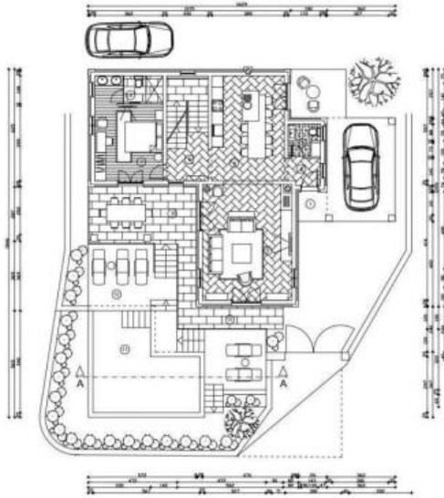
TLOCRT PRIZEMLJA M 1:100
