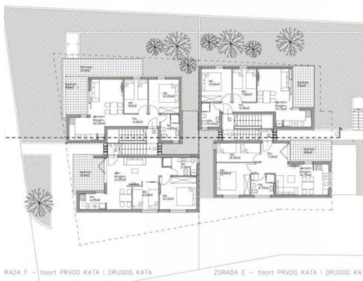
ZGRADA E – tloort PRIZEMLJA I PRVOG KATA
